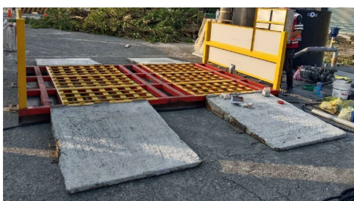
營建工地移動型洗車台實績(SCS20S323)
